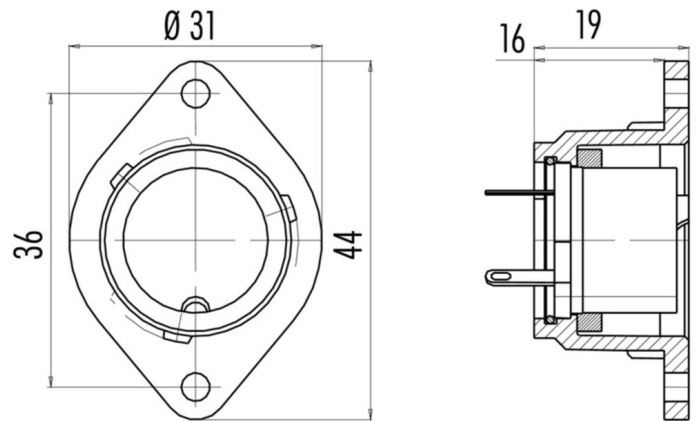
Ansicht ohne Polbild View without contacts
