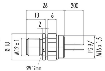
VA-Ausführung Stainless steel version
