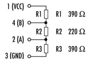
Schaltplan Wiring diagram
