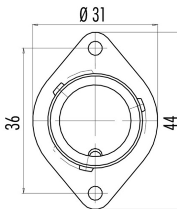
Ansicht ohne Polbild View without contacts
