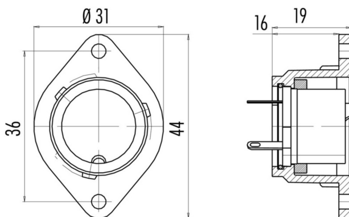
Ansicht ohne Polbild View without contacts
