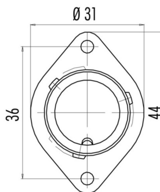
Ansicht ohne Polbild View without contacts
