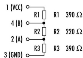
Schaltplan Wiring diagram
